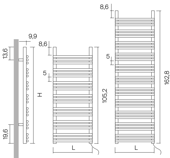
Elektrische Variante mit Thermostat und Fernbedienung Größen 105.20 x 48.50 cm mit 400 Watt 162.80 x 48.50 cm mit 600 Watt
